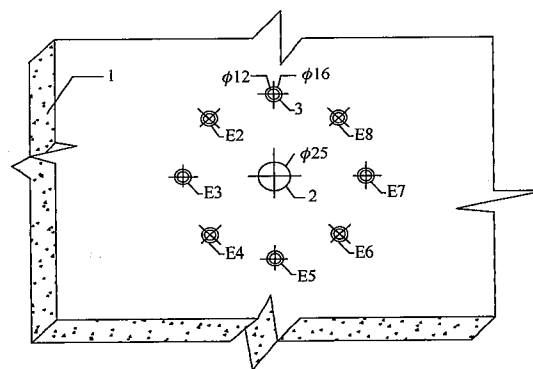
图1 后装式锈蚀传感器安装布局示意
